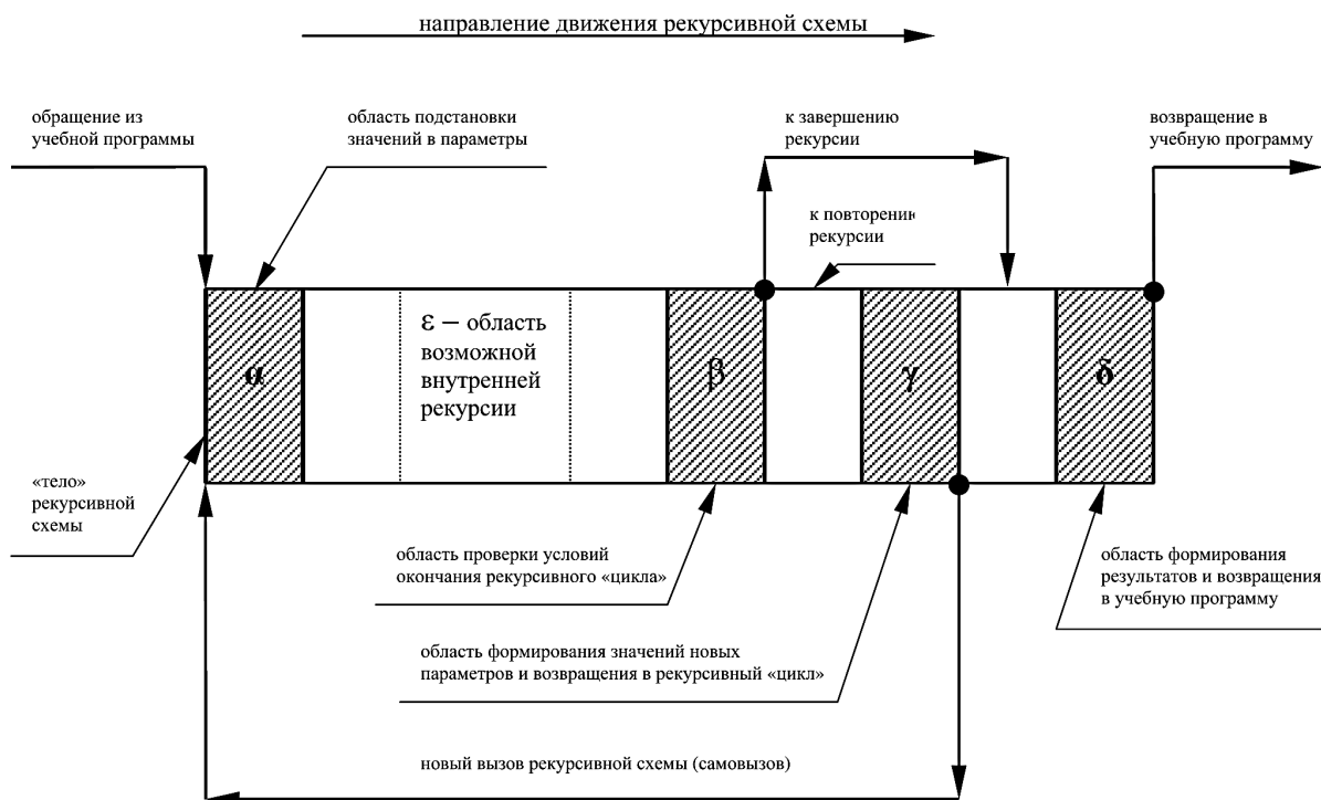
Рис. 1. Формальная структура «тела» рекурсивной схемы
