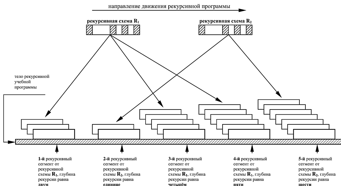
Рис. 2. Функциональная структура рекурсивной учебной программы
